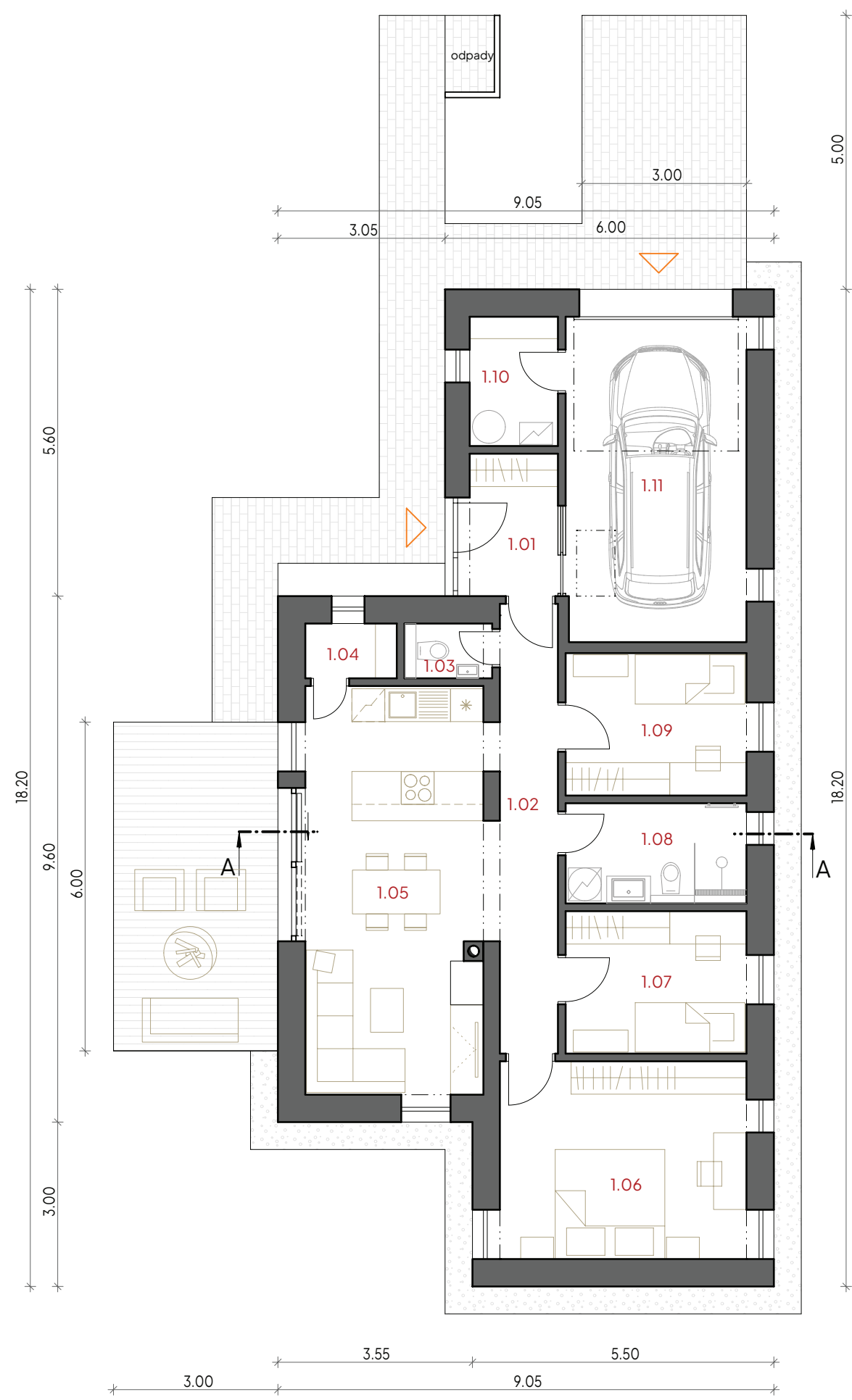
Pôdorys 1.NP
